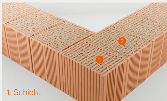
Eckverband für Wanddicke d = 30,0 cm
